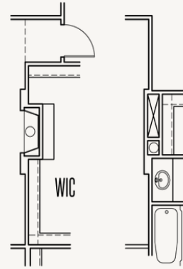
Optional Fireplace
